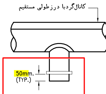
انشعاب ۹۰ درجه
