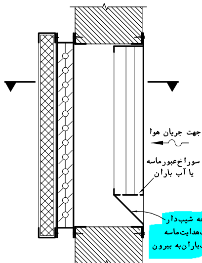
دریچه ماسه گیر با پره های قائم-مقطع قائم
