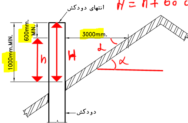
شکل ۶- عبور دودکش از سقف شیب دار
