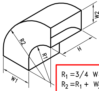
شکل ۴- زانوی تبدیل دوردار
