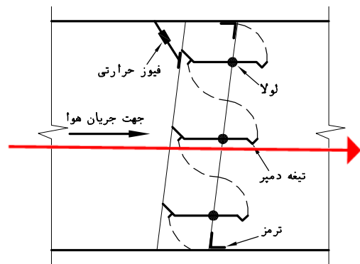
شکل ۳- دمپر آتش چند تیغه‌ای
