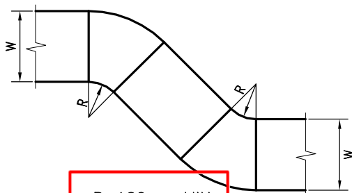
R=100\text{mm.MIN.}
