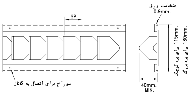
شکل ۳- قاب نگه‌دارنده پره‌های هدایت‌کننده هوا
