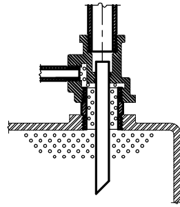
جداکننده هوا برای نصب روی دیگ
