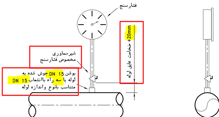
نصب فشارسنج روی لوله افقی
