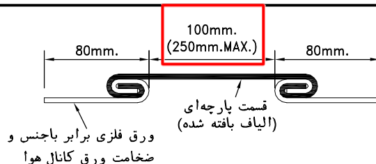
۱-مقطع قطعه قابل انعطاف
