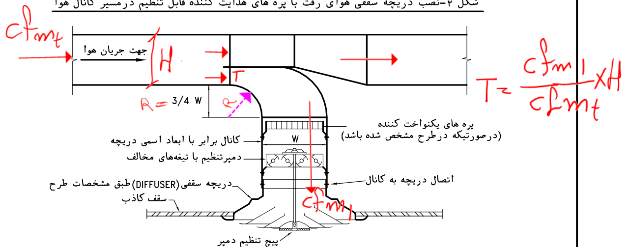
شکل ۳- نصب دریچه سقفی هوای رفت با انشعاب موازی از کانال هوای رفت
