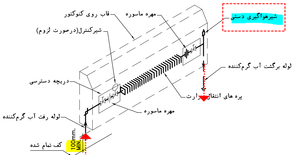
دیگرام لوله کشی کنوکتور در حالت تغذیه از پایین (UP-FEED CONNECTION)
