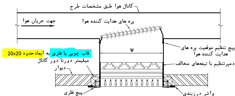
شکل ۲- نصب دریچه دیواری هوای رفت با پره های هدایت کننده قابل تنظیم در مسیر کانال هوا
