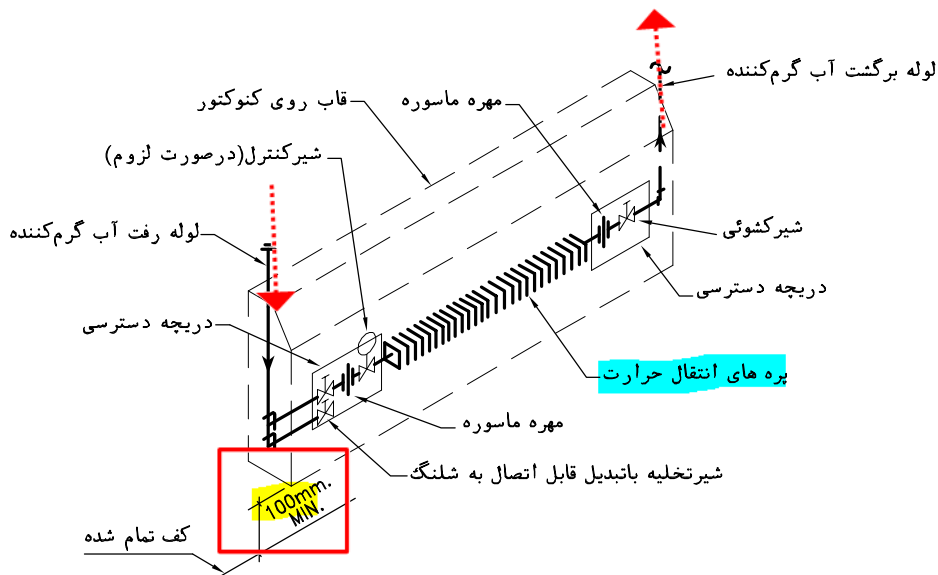
دیگرام لوله کشی کنوکتور در حالت تغذیه از بالا (DOWN-FEED CONNECTION)
