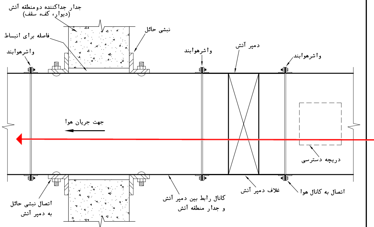
نصب دمپر آتش در مجاورت جدار جداکننده دو منطقه آتش
