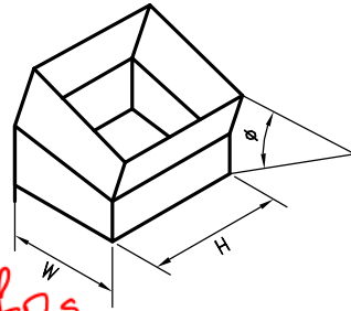
شکل ۵- زانوی مورب
