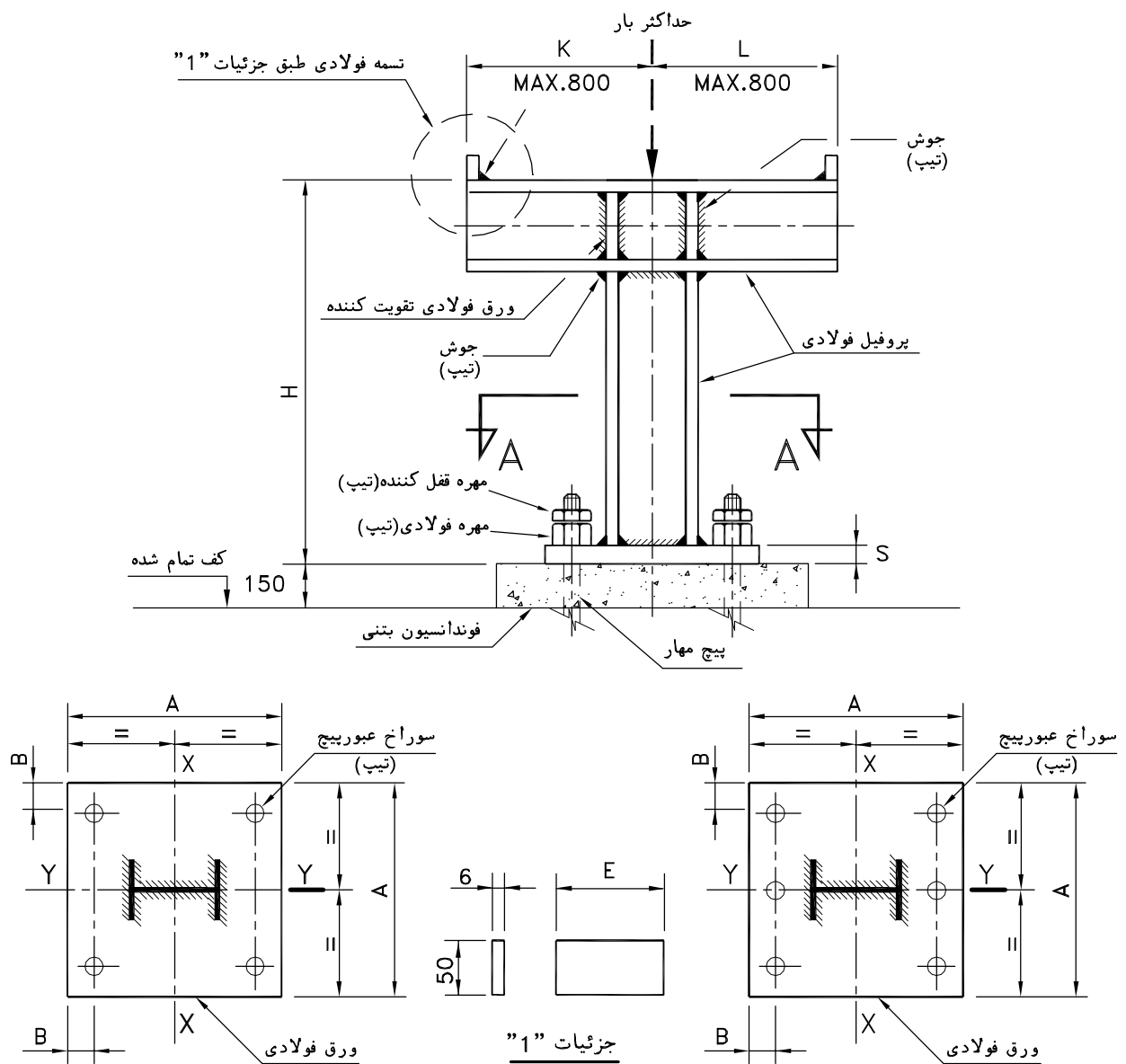
مقطع A-A برای تکیه گاههای شماره ۳ و ۱
