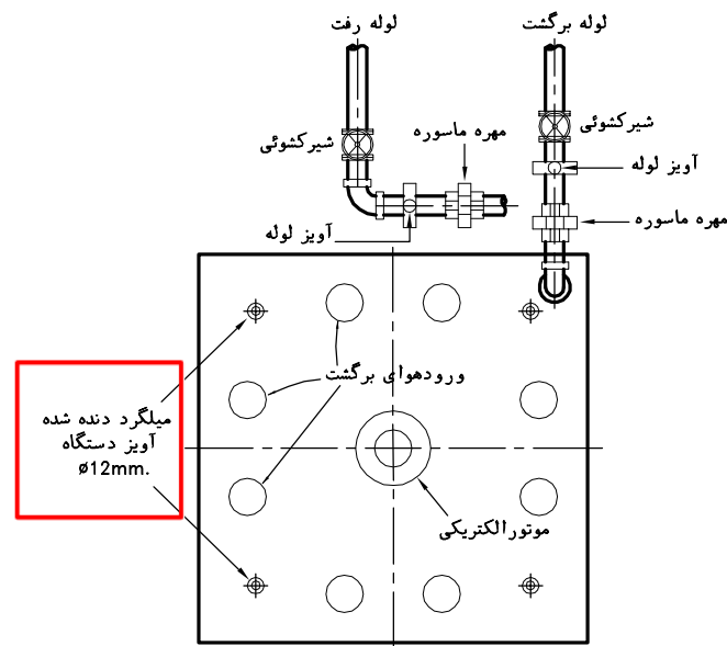
پلان
