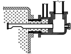
جداکننده هوا برای نصب روی دیگ
