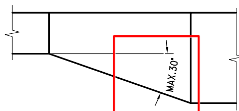
تبدیل نامتقارن
