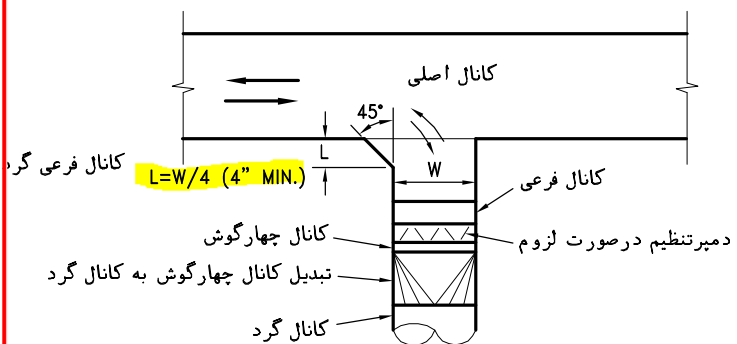
انشعاب کانال گرد از کانال چهارگوش
